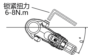
(图6)束仔螺丝锁紧扭力
