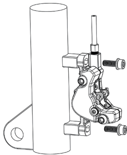
(图5)前叉安装
